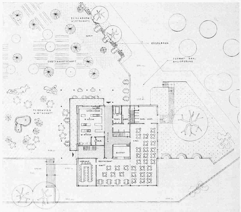
Erdgeschossgrundriss 1:600
