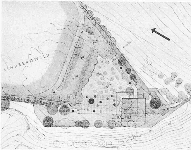
Lageplan 1:2000
