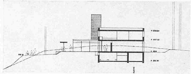
Schnitt 1:600
