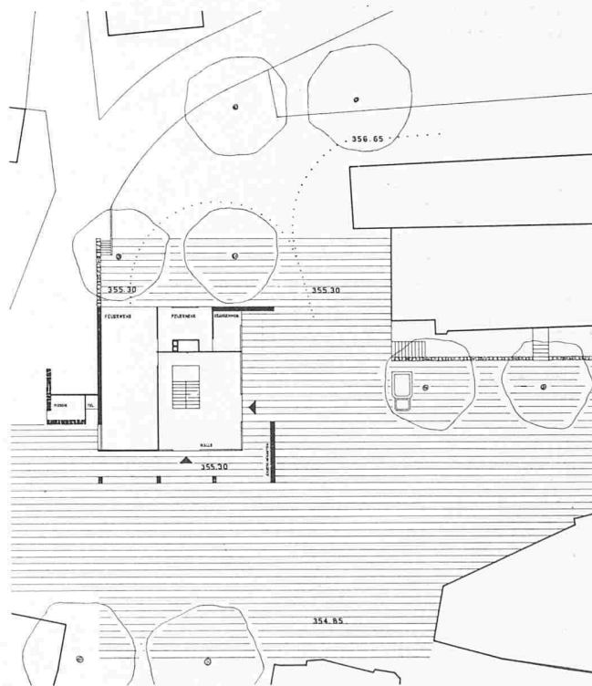
Erdgeschoss Masstab 1:600
