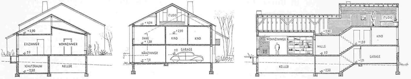
QUERSCHNITT WESTBAU
