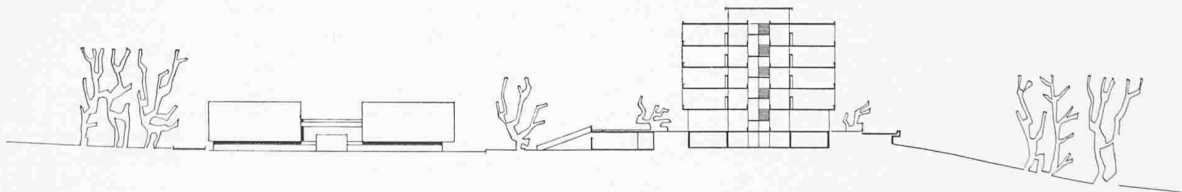
SÜD - WEST - ANSICHT TURNHALLEN
