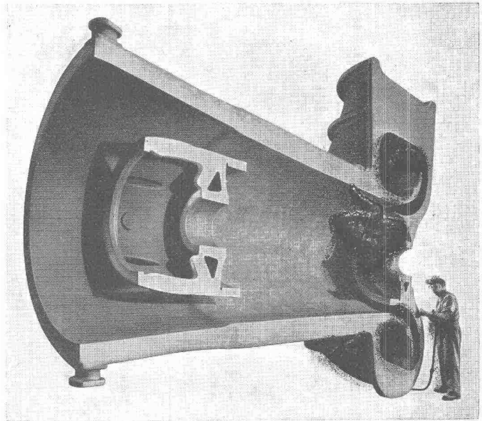
Oberteil zu einem Axialgebläse
