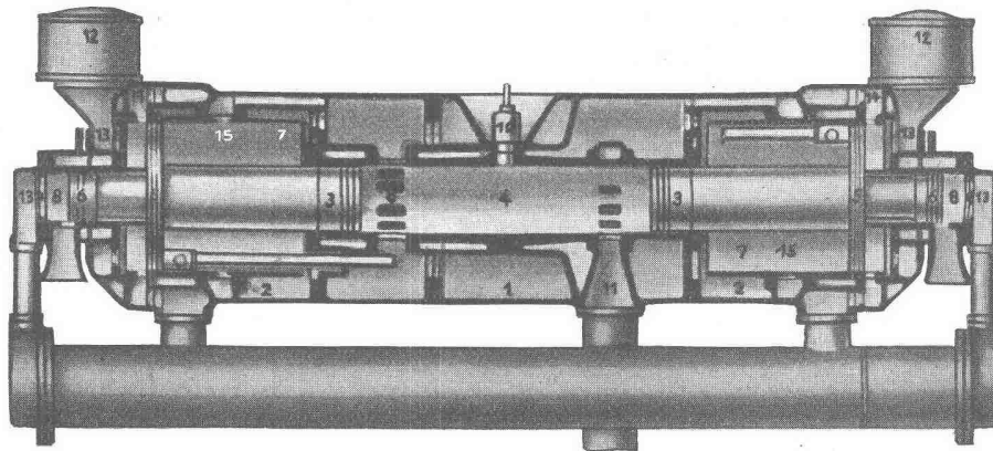
Schnittbild eines 2stufigen Junkers-Freikolben-Dieselmotors
