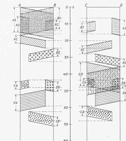
Bild 7. Gleiche Kreuzung und gleiche Betriebsweise, jedoch mehr Fahrspuren in den Zufahrten. Vorher mussten zum Beispiel A—B und A—D vereinigt bleiben. Jetzt sind sie getrennt und laufen gleichzeitig
