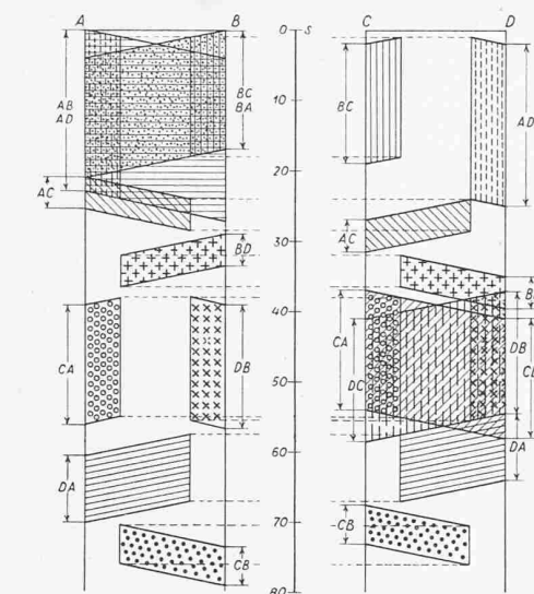
Bild 6. Zeit-Weg-Diagramm der einfachen Kreuzung mit Vier-Phasenbetrieb. Die Längsverbindung A—B und die Querverbindung C—D sind nebeneinander dargestellt. Abbiegende Verkehrsströme C—D sind beiden Seiten zu erkennen, z. B. ganz unten die Linksabbieger CB, die zuerst die Verbindung C—D und dann die Verbindung A—B besetzen. Angenommene Geschwindigkeit innerhalb der Kreuzung 5 m/s. Waagrecht Weg, senkrecht Zeit. Fussgänger können die Fahrbahn A überschreiten, solange kein Fahrzeug von oder nach A fährt.
