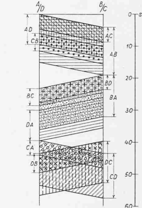
Bild 8. Einfache Kreuzung mit Drei-Phasenbetrieb. Andere Darstellung: Die Längsverbindung und die Querverbindung sind übereinander gezeichnet. Die Abbieger können leichter eingetragen werden. Eine Ungenauigkeit besteht darin, dass der Zeitaufwand der Rechtsabbieger ebensolang eingetragen ist wie derjenige der Linksabbieger. Diese vereinfachte Darstellung ist nur möglich, wenn die Wege A—B und C—D ungefähr gleich lang sind.
