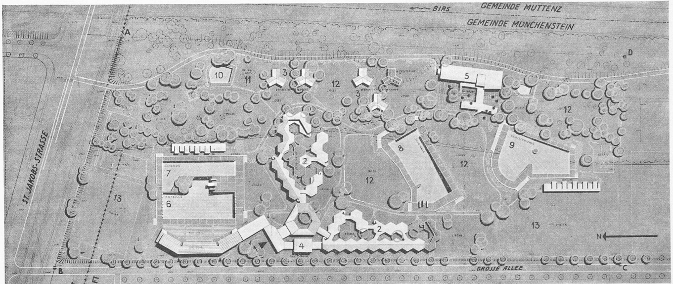
Lageplan, Masstab 1: 2500
