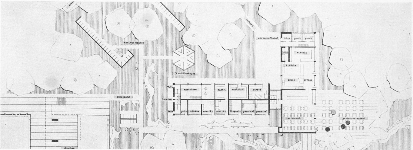
Erdgeschoss des Dienstgeb\u00e4udes mit Restaurant, Masstab 1:700
