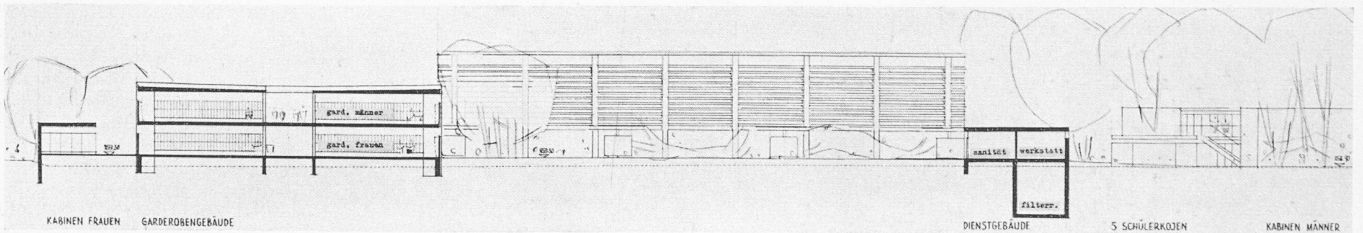
Schnitt West-Ost durch K\u00e4stchengarderobe und R\u00fcckansicht der Trib\u00fcne
