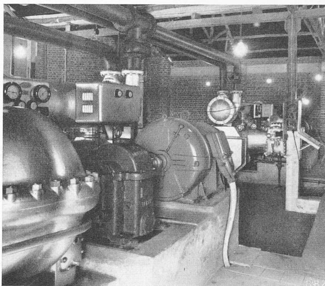
Bild 12. Inneres des Maschinenhauses mit zwei Carrier-Kälte-Kompressoren.
