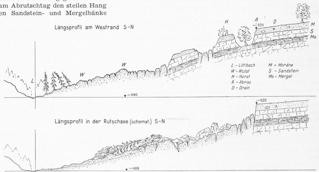
Der Bergrutsch von Notikon, Profile 1: 1000
