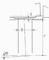
Bild 12. Die Spieländerung der Zentrierfläche einer um einen kleinen Winkel \alpha ausgelenkten Kupplung ist \Delta s = b \cdot \tan \alpha , Grössenordnung 20/1000 = 0,02 \text{ mm} .
