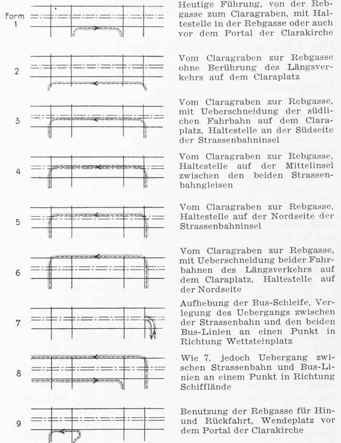
Bild 2b. Mögliche Führung der Buslinien (schräffelt)
