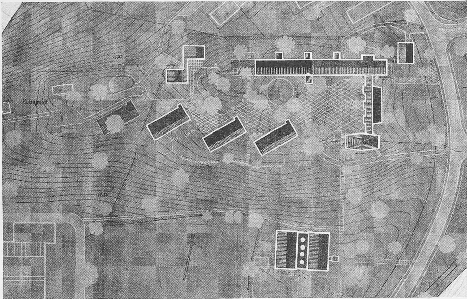
Lageplan 1:2500
