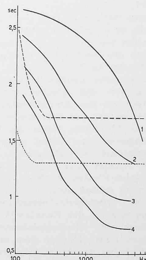
Bild 6. Tor und Vorhang offen. Gemessene Nachhallzeiten, Legende im Text
