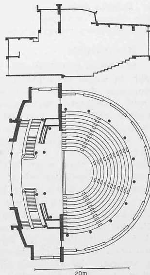
Bild 4. Bronzetor offen
