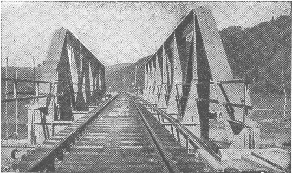
Tössbrücke Wila
