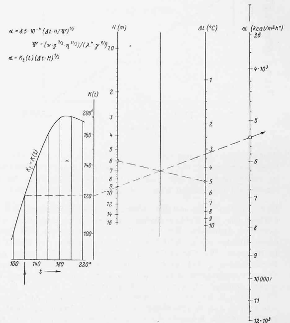
Bild 7. Nomogramm bei turbulentem Abfluss. Eingezeichnetes Beispiel: Wasserdampf, vertikales Rohr, turbulenter Film, H = 6 m, \Delta t = 50 °C, t = 120 °C gibt \alpha_m = 5400 kcal/m 2 h° C. Bei irrtümlicher Benützung von Bild 6 würde man erhalten \alpha_m = 5000 kcal/m 2 h° C.
