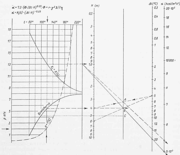
Bild 6. Nomogramm bei laminarem Abfluss. Eingezeichnetes Beispiel: Wasserdampf, vertikales Rohr, laminarer Abfluss, H = 4 m, \Delta t = 50 °C, t = 200 °C gibt \alpha_m = 5300 kcal/m 2 h° C.
