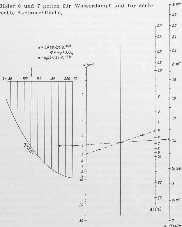
Bild 8. Nomogramm für Wasserdampf für liegende Rohre mit laminarem Abfluss. Eingezeichnetes Beispiel: Wasserdampf, horizontales Rohr, laminarer Film, d = 50 mm, \Delta t = 50 °C, t = 180 °C gibt \alpha_m = 12 200 kcal/m 2 h° C.
