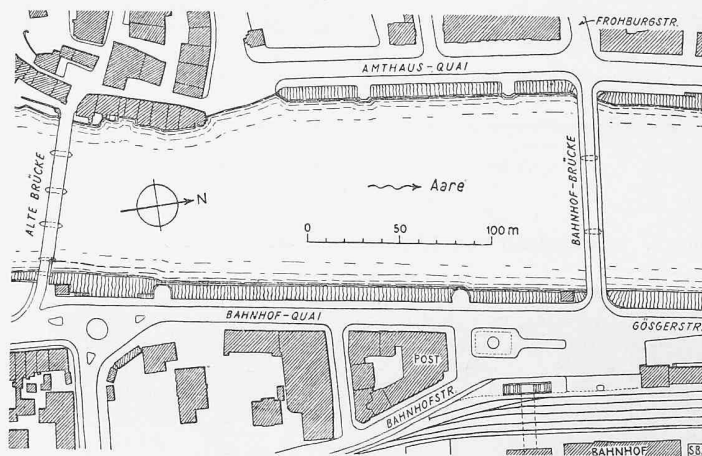
Bild 1. Lageplan, Masstab 1:4000
