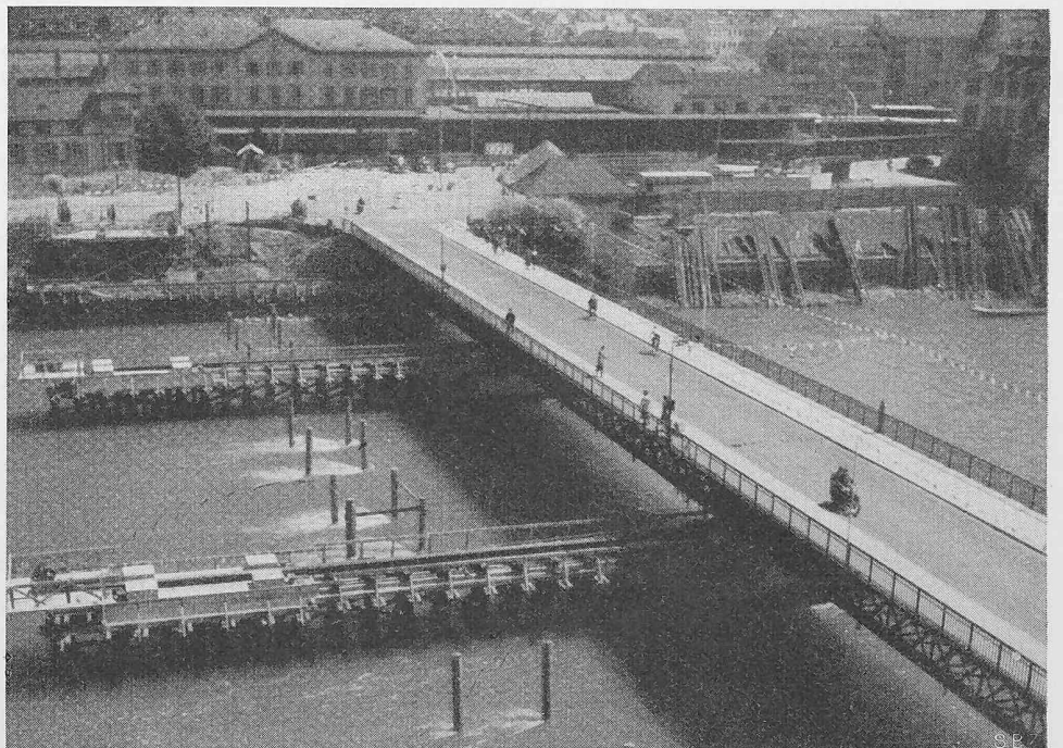
Bild 6. Die Brücke vor der Verschiebung
