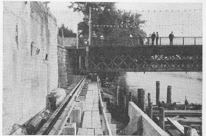
Bild 5. Verschubbahn vor dem linken Widerlager
