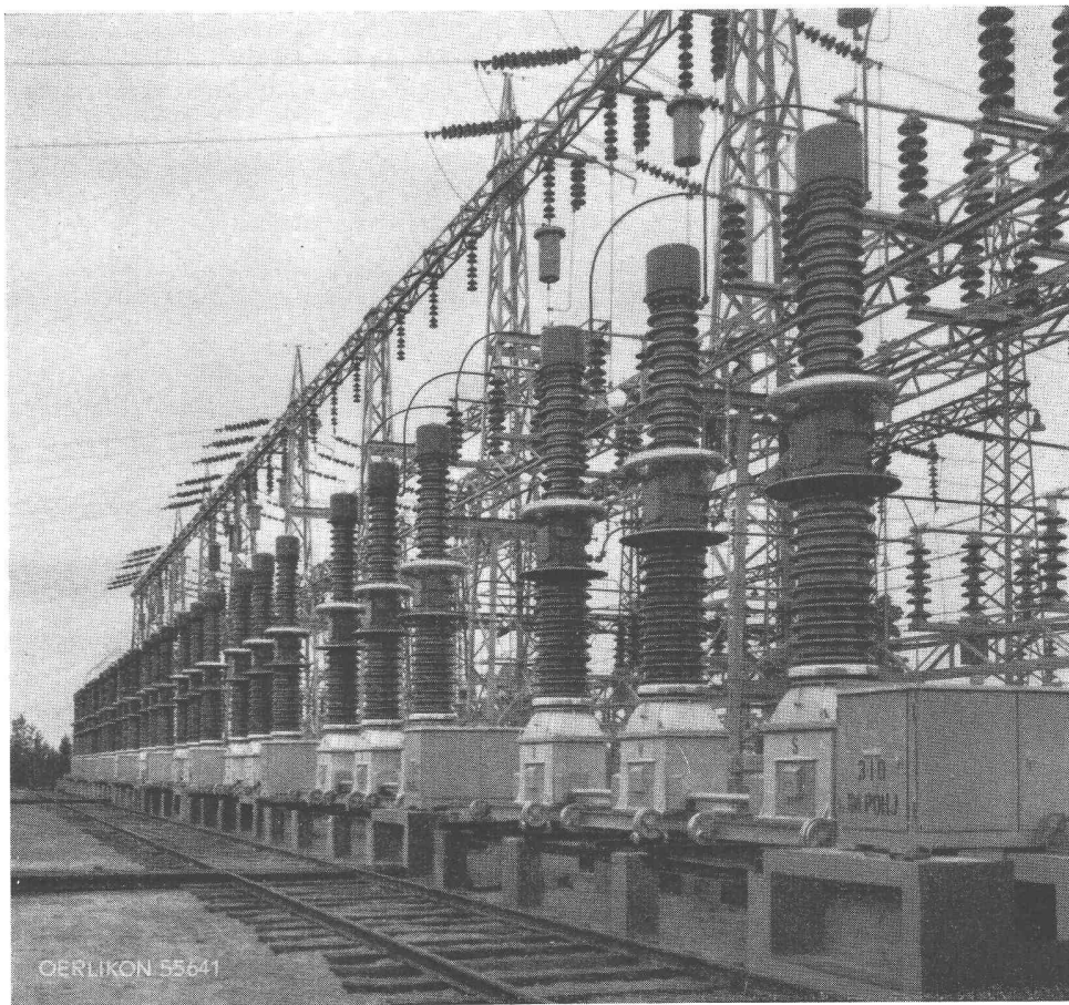
Gruppe von 9 ölarmen Schaltern, Typ TOF, 135 kV, 2500 MVA, in einer Transformatorstation in Finnland.
