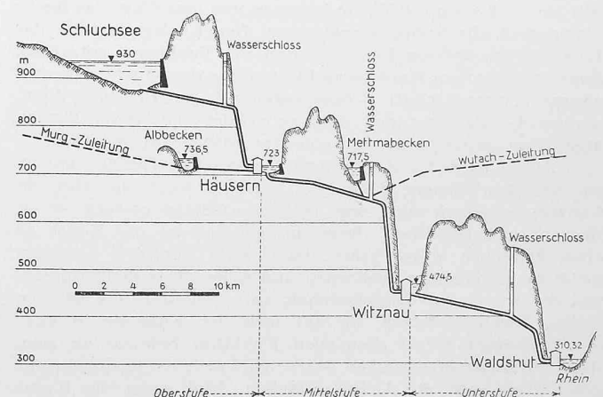
Bild 2. Längenprofil, Längen 1:450 000, Höhen 1:14 000
