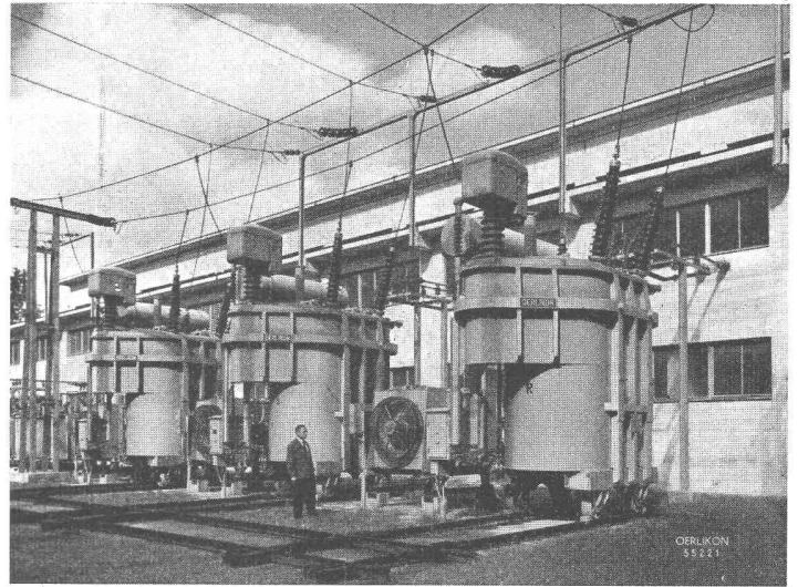
Drei Einphasentransformatoren, 38 000 kVA, Nennspannung 150/50/8 kVA, in Gruppe, von der Oberspannungsseite aus gesehen. Kraftwerk Benzau.
