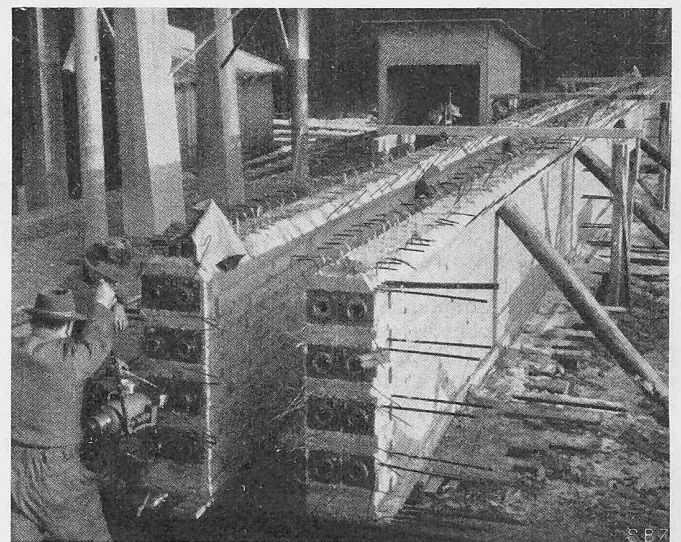
Bilder 19 und 20. Brücke über das Hilfswehr des Kraftwerks Wildeg-Brugg, Vorgespannte Trägerrippen 0,41 \times 1,2 m, als vorfabrizierte Träger am Ufer hergestellt. Total 4 Oeffnungen mit je 23 m Spannweite. Projekt: Ing.-Bureau E. Schübiger, Zürich.
