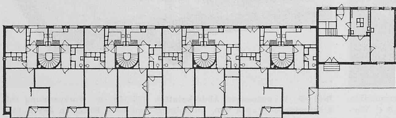
Bild 24. Gentofte. Erdgeschossgrundriss 1:500.
