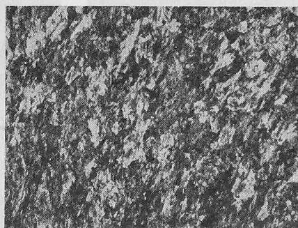
Bild 15. Mikrogefüge im aufgestauchten Kopf des pat., gez. Stahldrähtes
