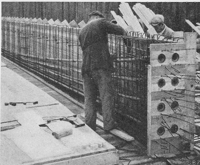
Bilder 19 und 20. Brücke über das Hilfswehr des Kraftwerks Wildeg-Brugg, Vorgespannte Trägerrippen 0,41 \times 1,2 m, als vorfabrizierte Träger am Ufer hergestellt. Total 4 Oeffnungen mit je 23 m Spannweite. Projekt: Ing.-Bureau E. Schübiger, Zürich.
