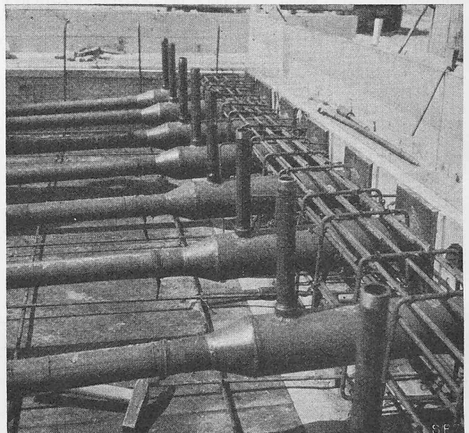
Bild 7. Vorspannarmierungen der Brücke Bild 6 mit Unterlagplatten und Uebergangsröhren und ihren Injektionsstutzen
