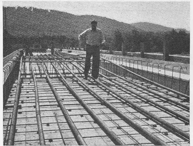
Bild 6. Vorspannarmierungen 80 t in einer Strassenbrücke verlegt
