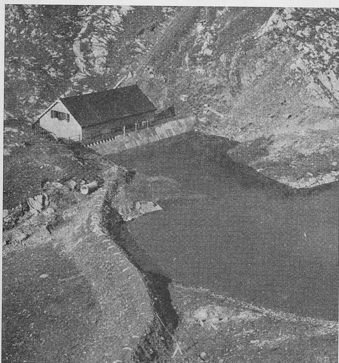
Bild 4. Das Pumpenhaus an der Saufila; im Vordergrund der Damm mit Zuleitung des Westarmes
