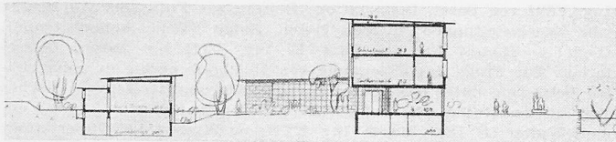
Schnitt durch Hauswirtschaft und Spezialraumtrakt
