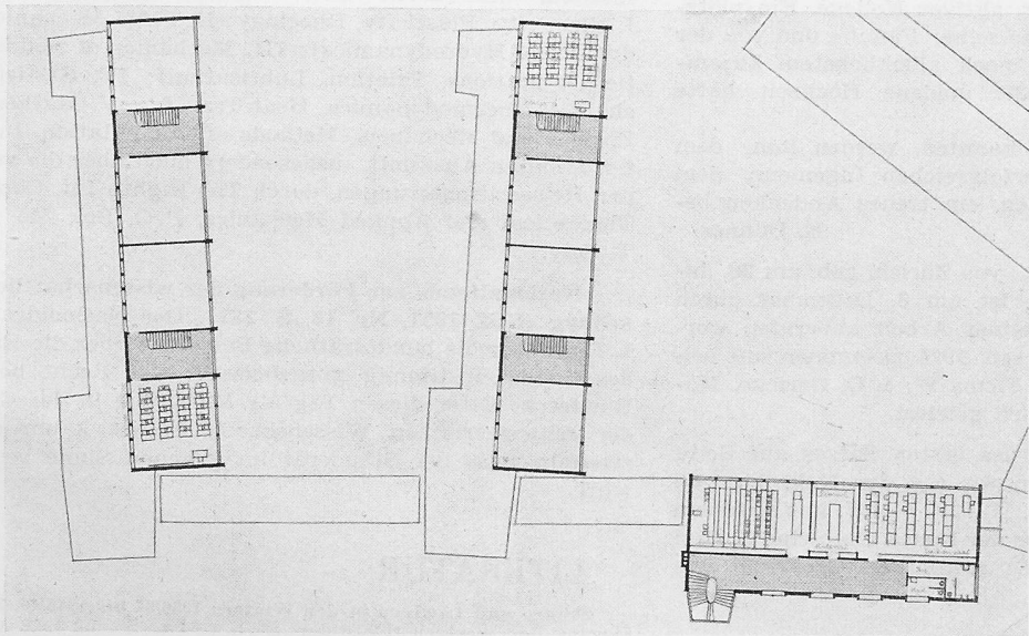
Obergeschoss-Grundriss 1:800
