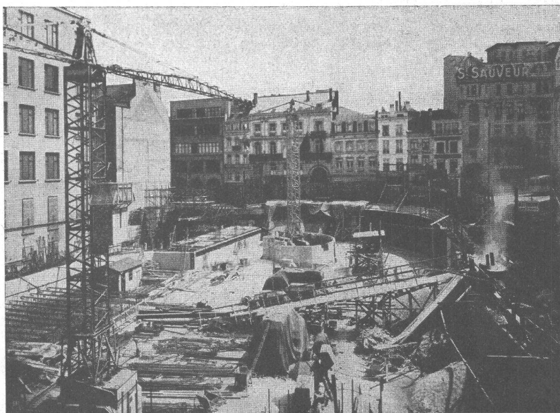
Caisse Générale d'Épargne et de Retraite, Bruxelles — A. Chambon, Architecte — L. M. Chapeaux, Ingénieur — S. A. Entreprises Louis de Waele — Grundwasserisolierung: ca. 5000 m 2
