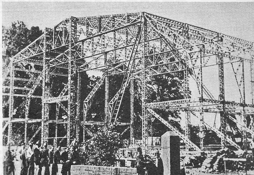
Bild 24. Demontierbare Theaterhalle in Duraluminium
