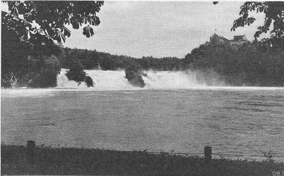
Bild 6. Der Rheinflall bei grosser Wasserführung, 5. Juli 1951, Wasserspiegel im Becken auf Kote 359,12 entsprechend dem vorgesehenen Winterstau, Wassermenge etwa 765 m 3 /s
