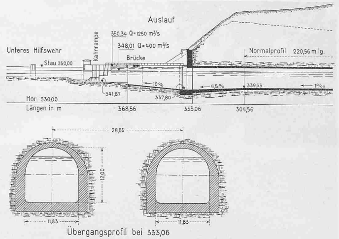
Bild 10a. Schnitt durch Stollen; Auslauf und unteres Hilfswehr, Masstab 1:2000; Übergangprofil Masstab 1:800
