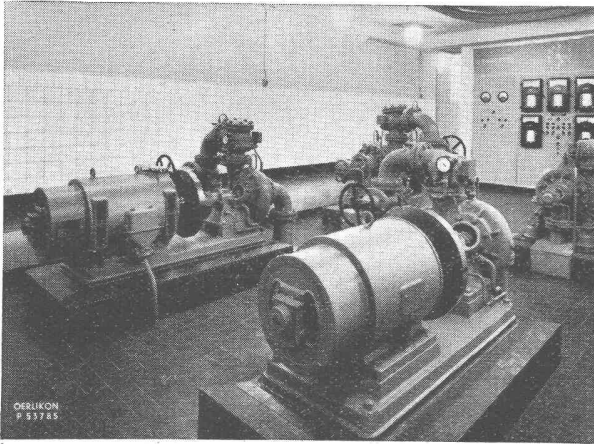
Trinkwasser-Pumpstation Calvaire bei Lausanne, ausgerüstet mit total drei Oerlikon-Combimotoren für 35, 55 und 75 PS.
