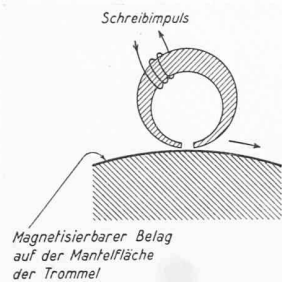
Bild 10. Magnetkopf für den magnetischen Speicher
