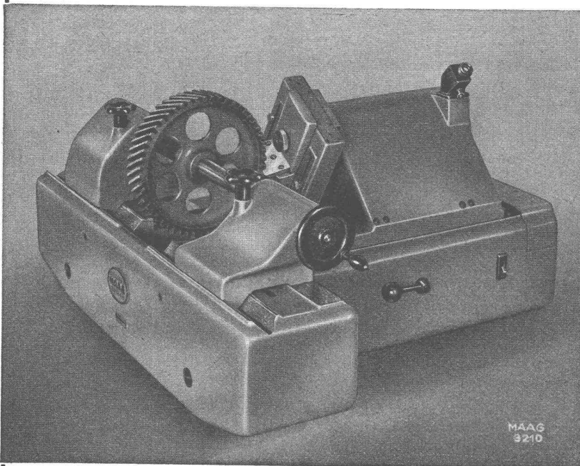
Zahnschräge-Messgerät Typ HM-30 für kleine Räder
