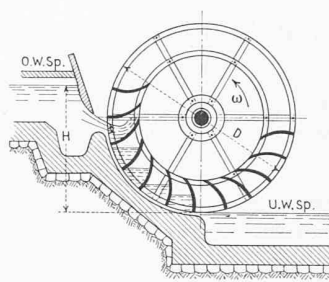
Bild 3. Mittelschlächt. Wasserrad
