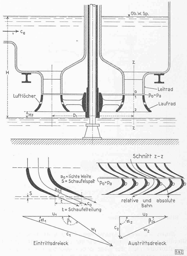
Bild 9. Girard-Turbine
