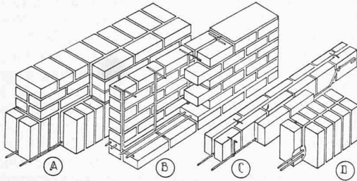
Bild 1. Armierte Ziegelbalken
