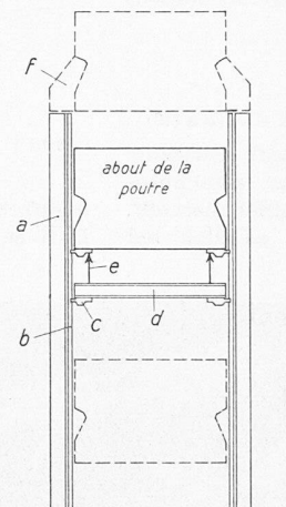
Fig. 15. Mise en place d'une poutre intérieure, 1:200. a poteau, b échelle de montage, c verrou, d traverse, e vérin, f dés d'appui
