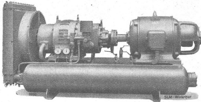
Luftgekühlter SLM-Chassis-Kompressor, Leistung 36 PS
