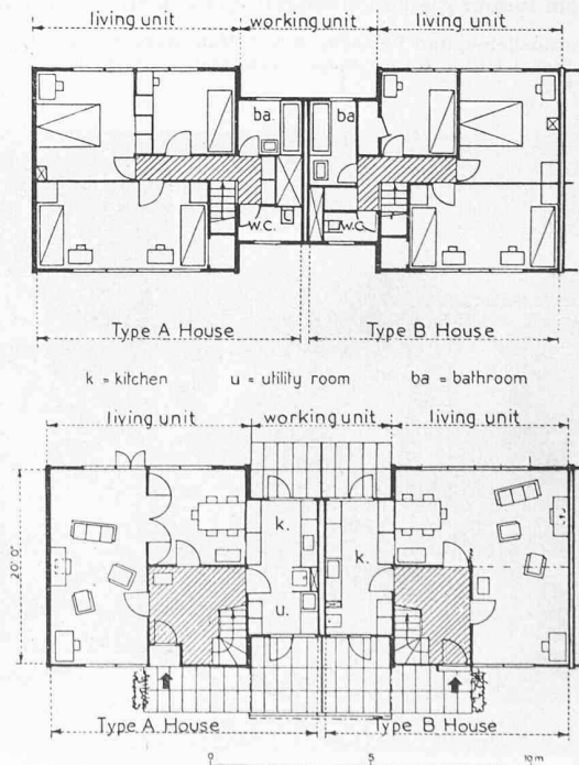
Bild 2. Howard-Haus, Erdgeschoss und Obergeschoss 1:250. Utility room = Putz-, Heiz-, Wasch- und Abstellraum
