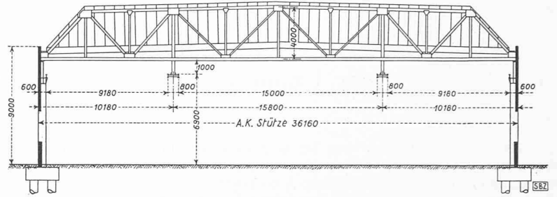
Bild 1. Automobil-Reparatur-Werkstattthalle, Querschnitt 1 : 400
