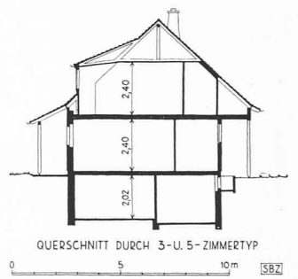
Bild 5. Schnitt 1:300
