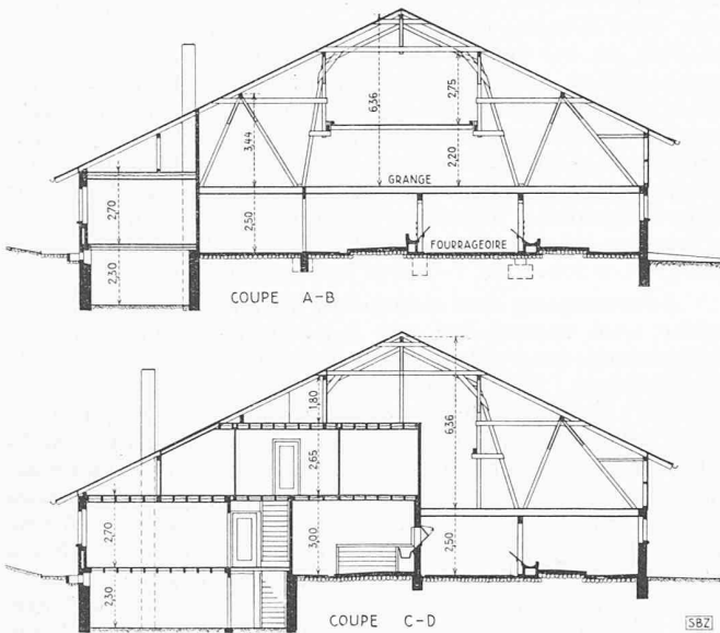
Fig. 4. Coupes 1:300
