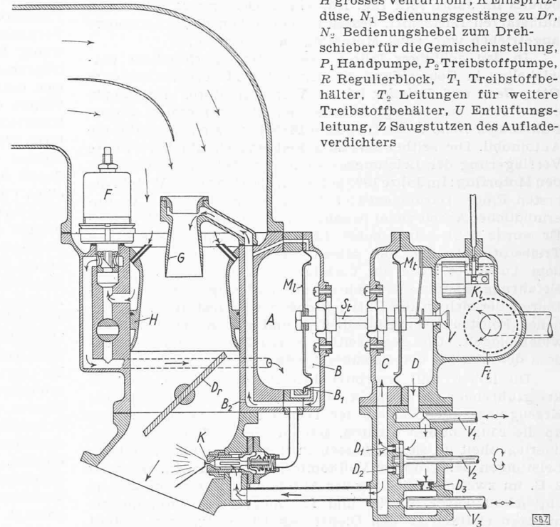
Bild 3. Schema der Regeleinheit der Stromberg-Einspritzvorrichtung. A u. B luftseitige Regelkammern, B1 u. B2 Blenden im Regelluftstrom, C u. D treibstoffseitige Regelkammern, D1 Düse für wirtschaftlichen Flug (mageres Gemisch), D2 id. (reiches Gemisch), D3 Düse für Hochleistung (sehr reiches Gemisch), Dr Luftdrosselklappe, F automatischer Gemischregler (beeinflusst Regelluftdruck in A ), F1 Treibstofffilter, G kleines Venturirohr, H grosses Venturirohr, K Einspritzdüse, K1 Entlüftungskammer, M1 Luft-Regelmembrane, M2 Treibstoff-Regelmembrane, St Regelstange, V Hauptregelventil, V1 Leerlaufschieber, V2 Drehschieber für wirtschaftlichen Flug (mageres oder reiches Gemisch), V3 Zuschaltventil für Hochleistung
