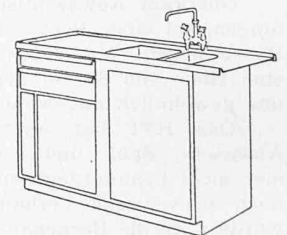
Bild 29. Spültisch-Einheit zur Küche von Bild 4. Unter dem Tropfbrett Besteckschublade. Masse: 130 x 60 x 85 cm
