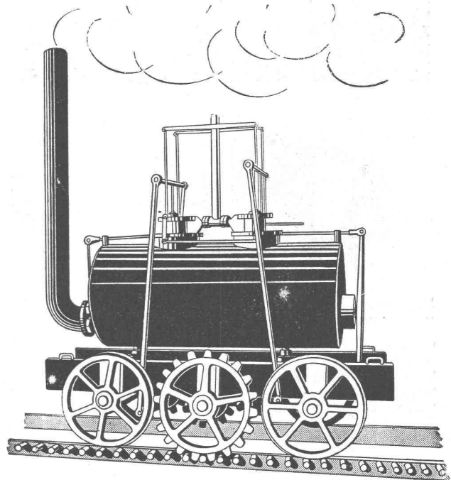
Lokomotive von Blenkinsop 1812, lief 5 km/St.
