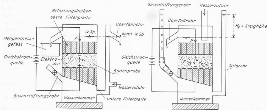
Bild 10a. Oedometeranordnung für Mengenmessung
