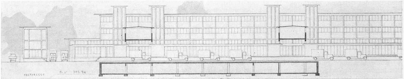
Oben: Querschnitt 1 : 600 durch Warenabteilung, Spedition und Garagen ; darunter Längsschnitt 1 : 600 durch Speditionshof
