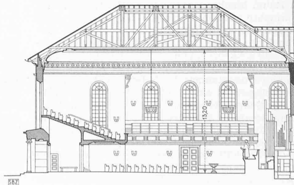
Bild 8. Längsschnitt 1 : 400
