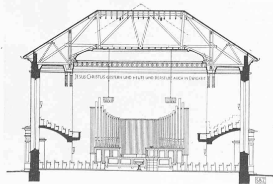
Bild 7. Querschnitt 1 : 400
