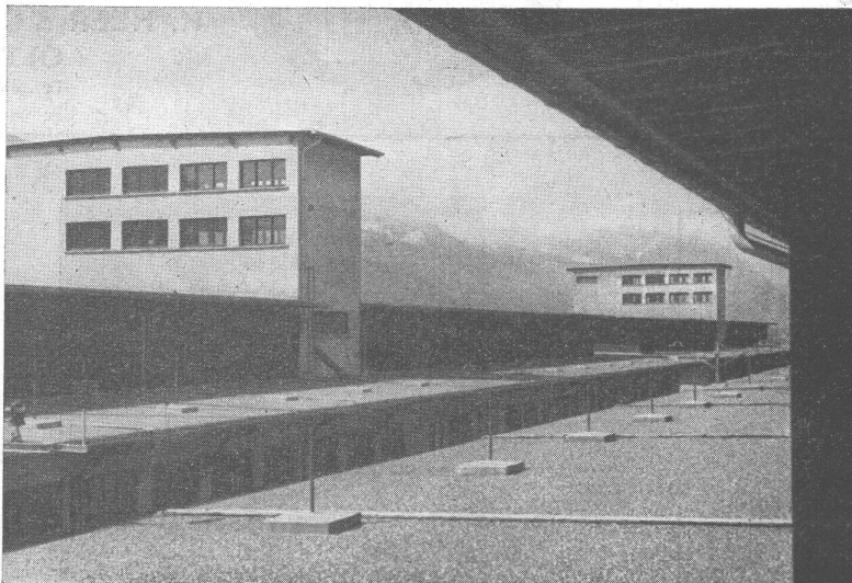
Ausführung der Kieslebedächer für 2 Getreidemagazine in Brunnen 5600 m 2
