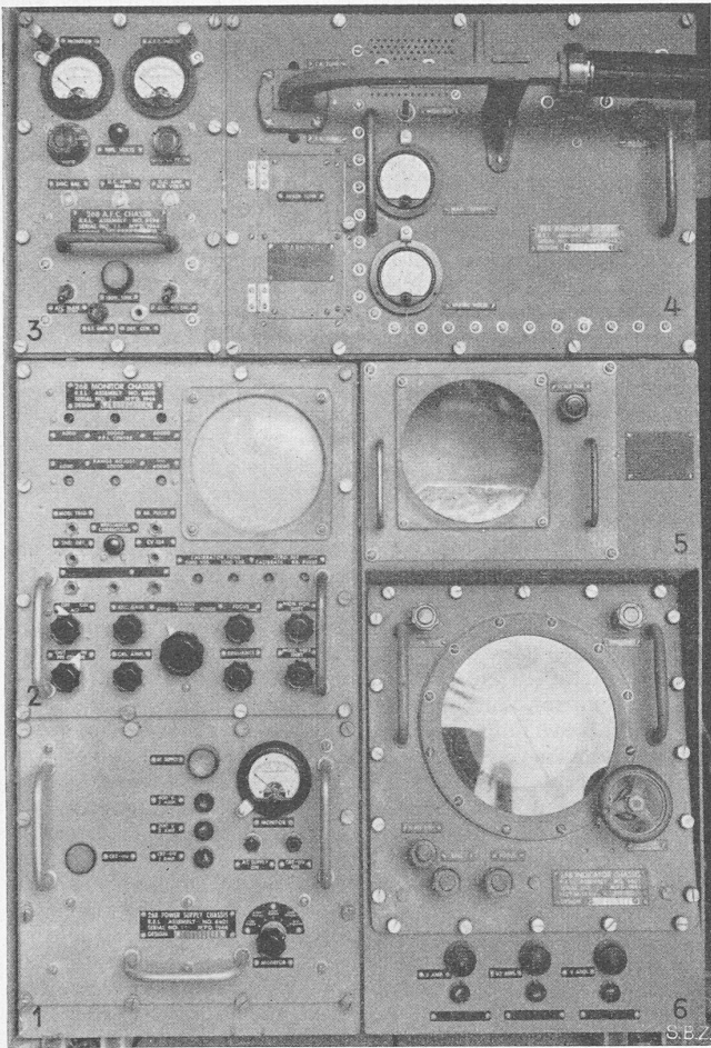
Bild 2. Vorderansicht des Gerätekastens. 1 Gleichrichter, 2 Impulsatz mit Kontrollröhre, 3 Stromlieferung und Frequenzkontrolle, 4 Sender-Empfänger mit Wellenleiter, 5 Behälter für Kompass (wird nur auf Schiffen verwendet), 6 P.P.I.-Röhre
