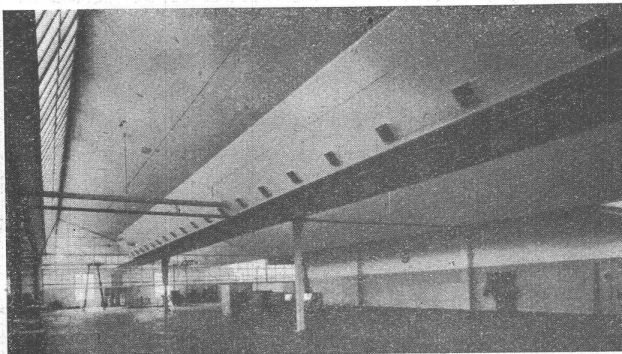
Ringspinnsaalverbreiterung in Aesch
