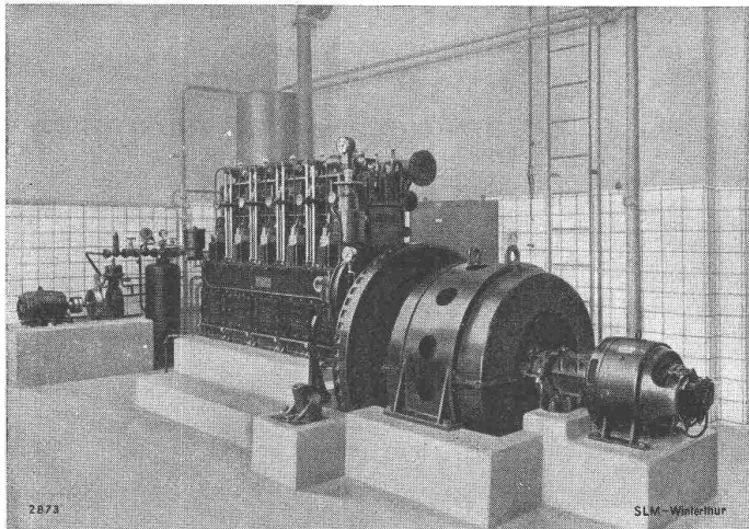
Vollautomatische Notstromanlage „SLM-Winterthur“ von 250 PS Leistung
