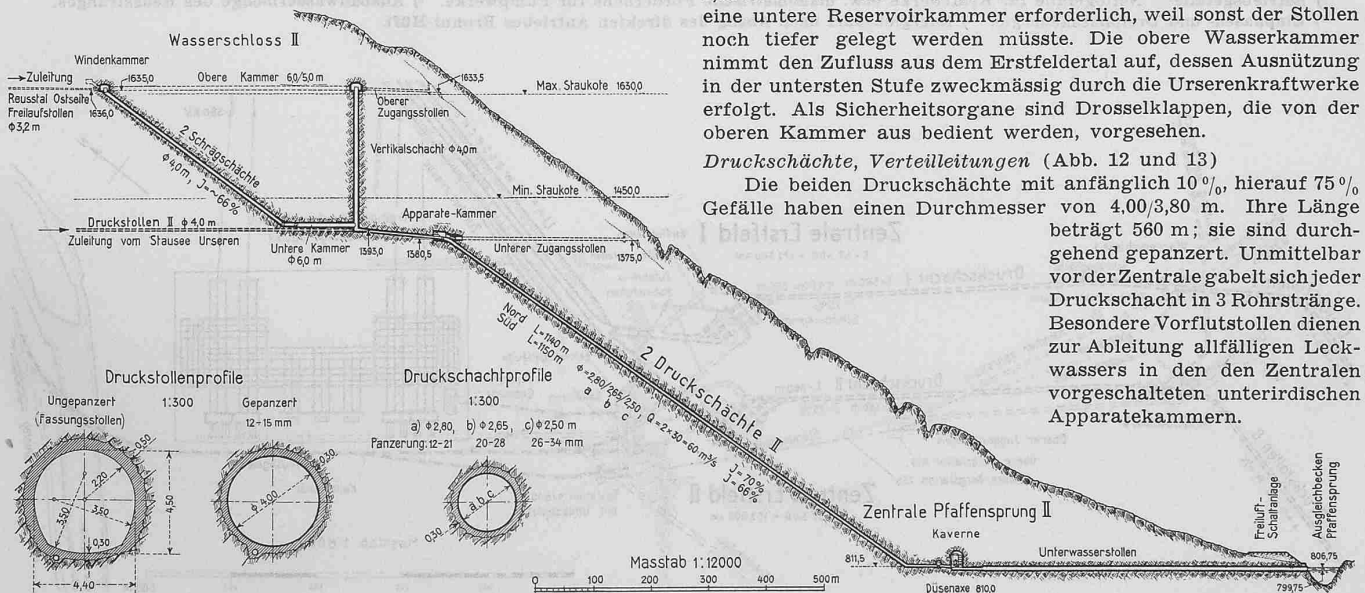
Abb. 10. Hauptkraftwerk Pfaffensprung II, Längenprofil Wasserschloss-Zentrale 1 : 12000 und Stollenprofile 1 : 300
