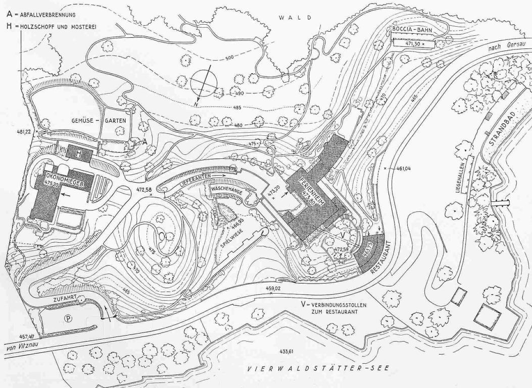
Abb. 1. Lageplan 1:2000
