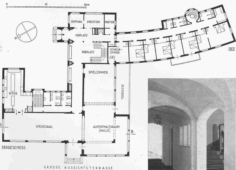
Abb. 10 und 11. Grundrisse 1 : 500
