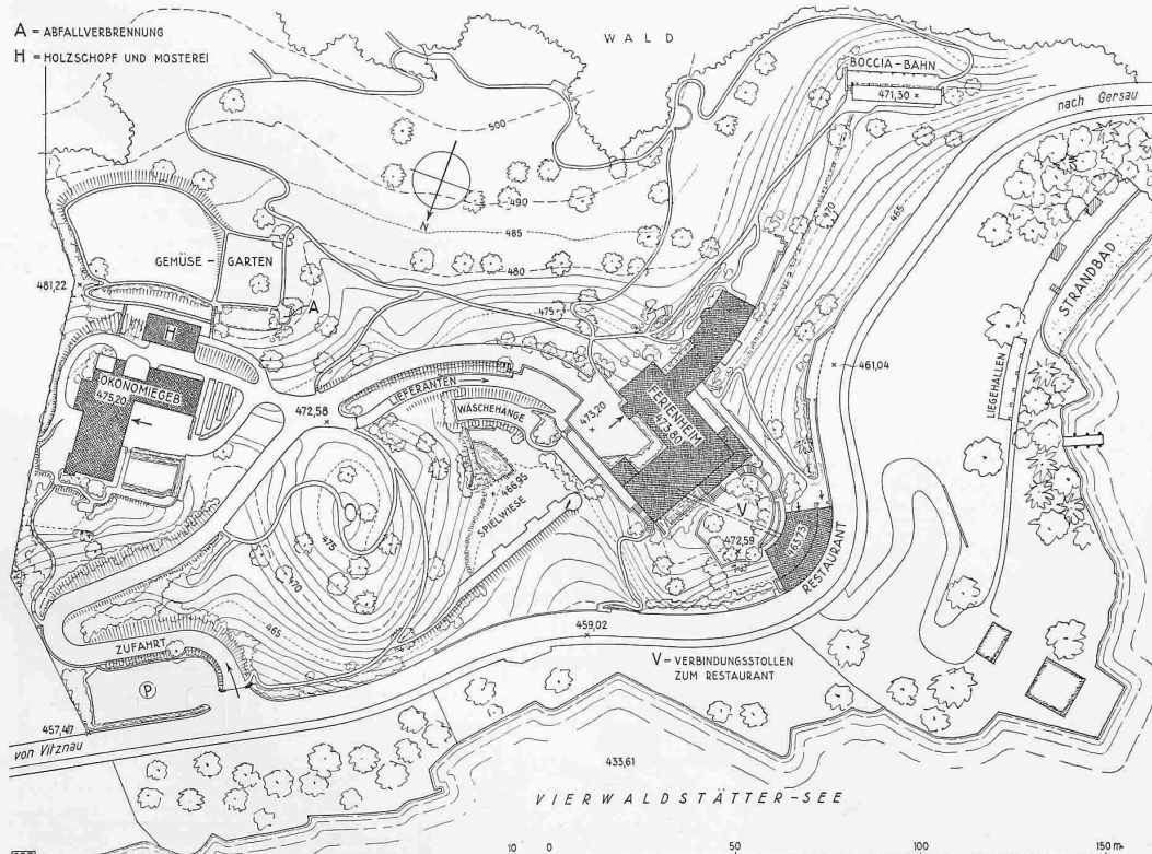
Abb. 1. Lageplan 1:2000
